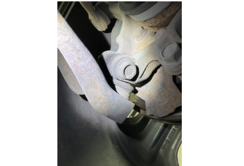
Direksiyon sistemi, Rot kolu/Rot başı, sol > Hasarlı
