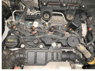
Komünikasyon/Navigasyon/EğlenceMotor, Motor üst kapağı, plastik sistemleri, Anten > Sökülmüş-Yok > Sökülmüş-Yok
