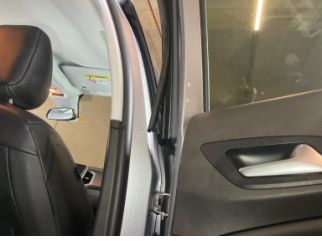
Kapı, sağ arka, Kapı fitili > Sabitlemesi Hatalı
