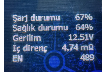
Elektrik donanımı/Pano, Akü > Test Sonucu
